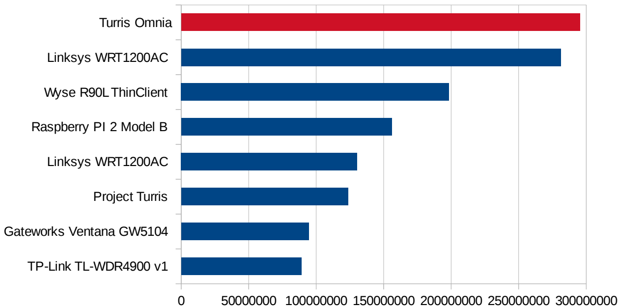
MD5 benchmark
